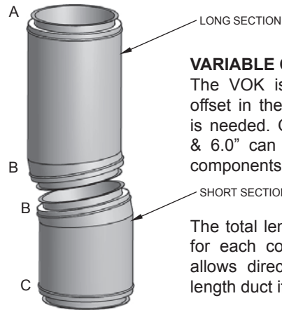
FIG. 28 - VOK CONFIGURATIONS
